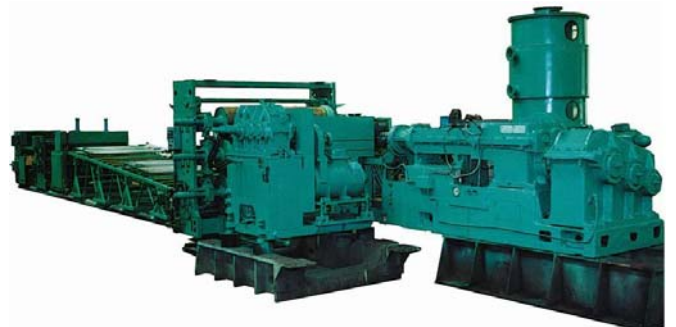
Лінія для виготовлення деревнополімерних листів ЛДПЛ-1200
