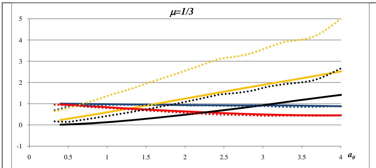
Figura 7.1.a: Comparación de los términos de las funciones de impedancia normalizadas del modelo tridimensional y plano calibrado según la propuesta de Luco y Hadjian [18] para \mu=1/3 .
