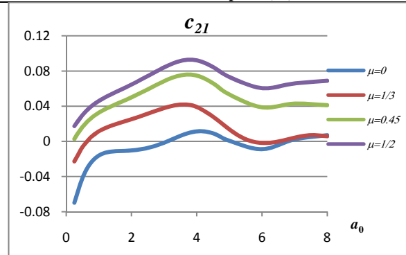
Figura 6.3.d: Parte imaginaria de la función de impedancia de translación y rotación acopladas ( c_{21} ).
