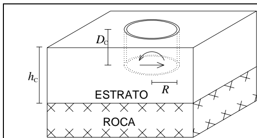
Figura 11.7.a: Modelo tridimensional para una cimentación circular enterrada en un estrato con paredes en total contacto en un estrato empotrado.
