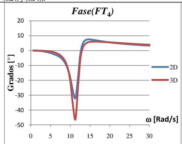
Figura 7.2.h: Fase de la función de transferencia entre el desplazamiento total en la base de la cimentación y el movimiento en superficie libre (ecuación (6.25) y (6.55)).
