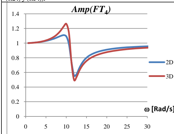
Figura 7.2.g: Amplitud de la función de transferencia entre el desplazamiento total en la base de la cimentación y el movimiento en superficie libre (ecuación (6.25) y (6.55)).
