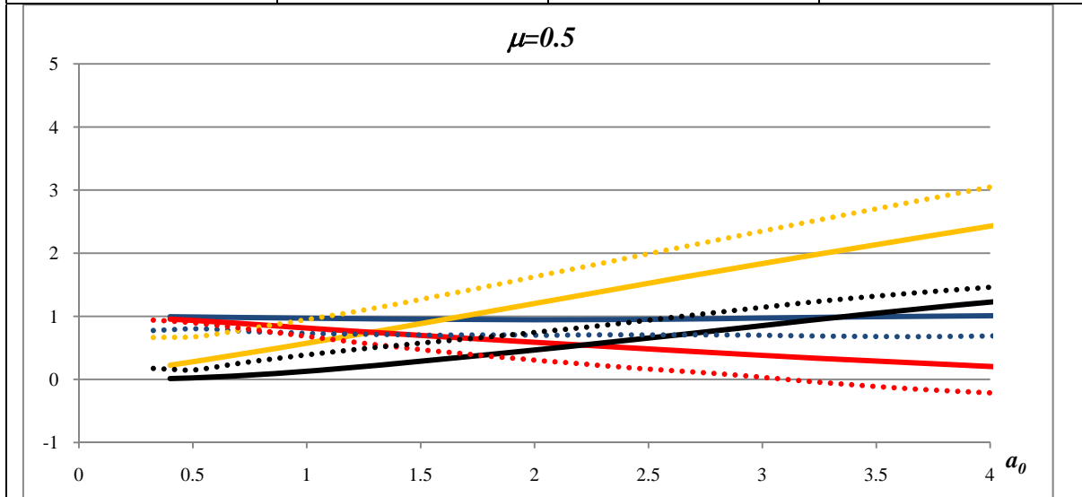
Figura 7.1.c: Comparación de los términos de las funciones de impedancia normalizadas del modelo tridimensional y plano calibrado según la propuesta de Luco y Hadjian [18] para \mu=0.5 .
