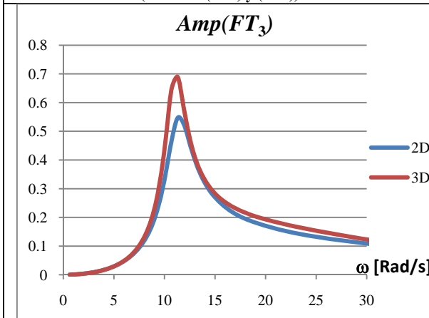
Figura 7.2.e: Amplitud de la función de transferencia entre el desplazamiento de la masa debido a la rotación de la cimentación y el desplazamiento en superficie libre (ecuación (6.24) y (6.54)).
