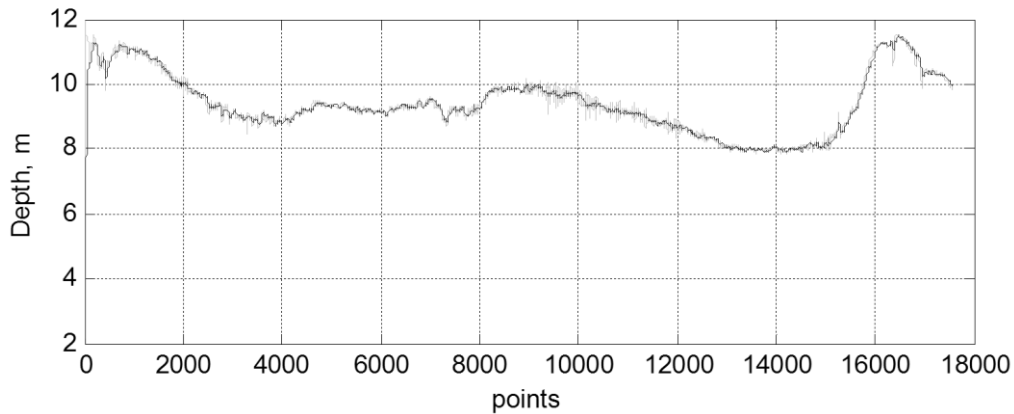
Рис. 2. Результат фільтрації даних глибини фільтром Калмана: — — вихідні (незашумлені) дані; — — фільтровані дані ( Q = 0,01 , R = 10 )
