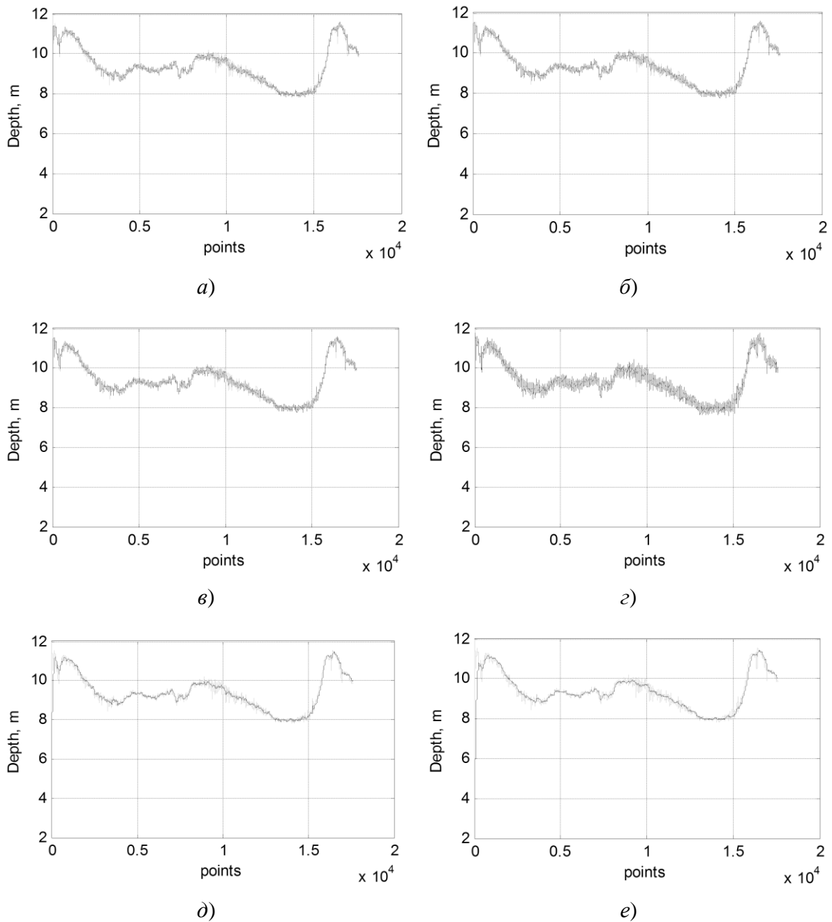
Рис. 3. Результат фільтрації даних глибини фільтром Калмана ( — — вихідні (незашумлені) дані; — — фільтровані дані): а) — Q=0,05 , R=10 ; б) — Q=0,1 , R=10 ; в) — Q=1 , R=10 ; г) — Q=0,01 , R=1 ; д) — Q=0,01 , R=20 ; е) — Q=0,01 , R=50
