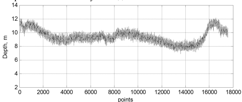
Рис. 1. Зашумлені дані
