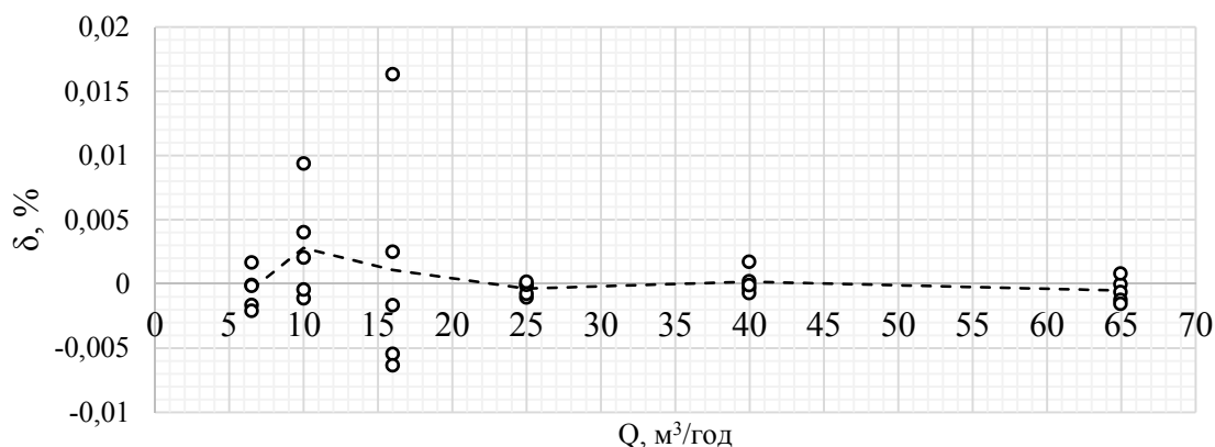
Рис. 6. Залежність величини додаткової \delta_{\Delta P} похибки від об'ємної витрати Q
