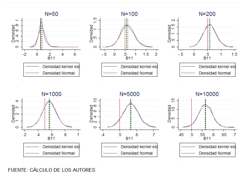
Gráfico 13. Modelo Multinomial estimado por Logit (proceso generador de datos t-student)
