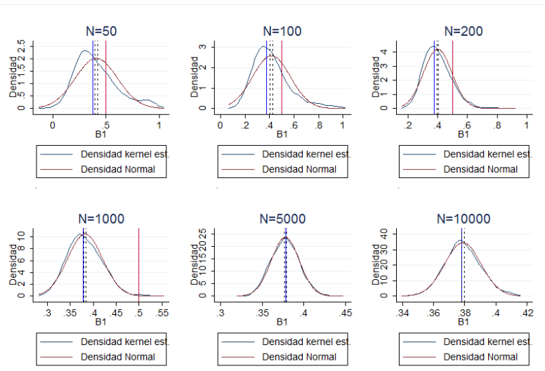
Gráfico 4. Modelo Condicional estimado por Probit (proceso generador de datos logístico)
