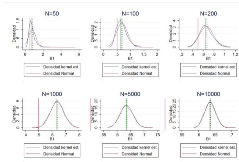
Gráfico 15. Modelo Condicional estimado por Logit (proceso generador de datos t-student)
