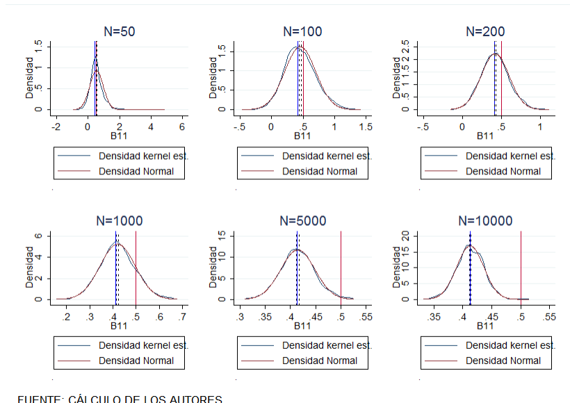
Gráfico 14. Modelo Multinomial estimado por Probit (proceso generador de datos t-student)
