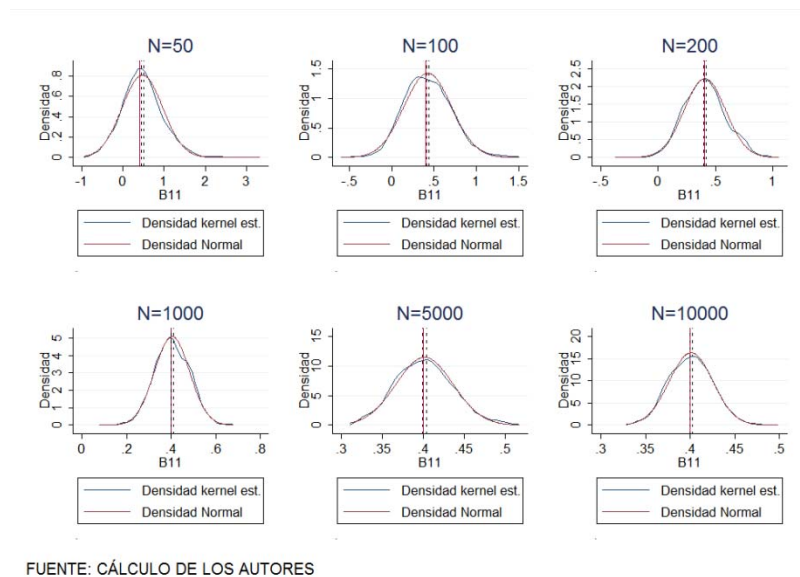
Gráfico 8. Modelo Multinomial estimado por Probit (proceso generador normal)
