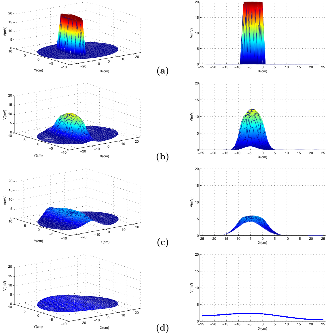
Figura 3.11 Solución al problema usando elementos finitos y siendo f igual a 0; (a) t = 0ms , (b) t = 1ms , (c) t = 3ms y (d) t = 38ms
