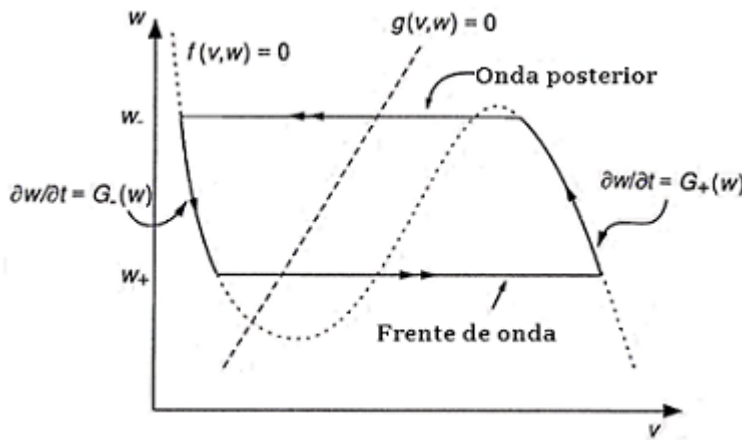
Figura 3.5 Dinámica para el sistema FitzHugh-Nagumo.
