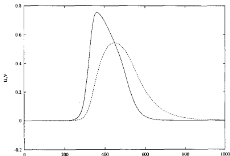
Figura 3.3 Forma de onda para el sistema FHN modificado.
