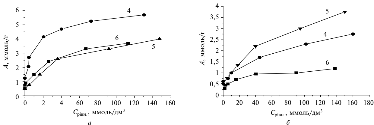
Рис. 8. Ізотерми сорбції фосфат-йонів сумішами \text{Al}(\text{OH})_3\text{-La}(\text{OH})_3 (4), \text{Al}(\text{OH})_3\text{-Ce}(\text{OH})_4 (5) і гідроксидом алюмінію (6) при pH = 2,4–2,6 (а) та pH = 8,9–9,1 (б)
