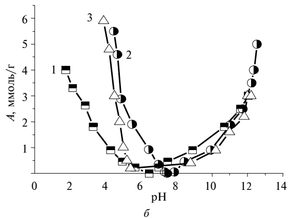
Рис. 4. pH розчинів HNO_3 і NaOH на фоні 0,1 М розчину NaNO_3 за наявності сорбентів (а) та залежність сорбційної ємності A від pH (б) для сумішей гідроксидів лантану і титану (зразки 1–3)
