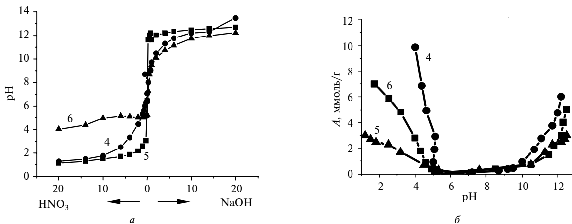
Рис. 7. Вимірювання pH розчинів \text{HNO}_3 і \text{NaOH} на фоні 0,1 М розчину \text{NaNO}_3 за відсутності та за наявності сорбентів (а) та залежність сорбційної ємності A від pH (б); 4 – \text{Al}(\text{OH})_3\text{-La}(\text{OH})_3 , 5 – \text{Al}(\text{OH})_3\text{-Ce}(\text{OH})_4 , 6 – \text{Al}(\text{OH})_3
