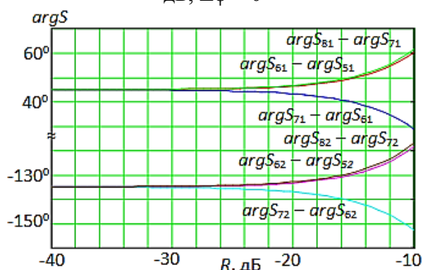
Рис. 8. Разность фаз между соседними выходами матрицы при возбужденні входів 1 і 2, I = -30 дБ, \Delta = 0 дБ, \Delta\varphi = 0
