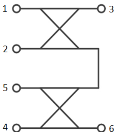
Рис. 3. Два каскадно соединенных НО
