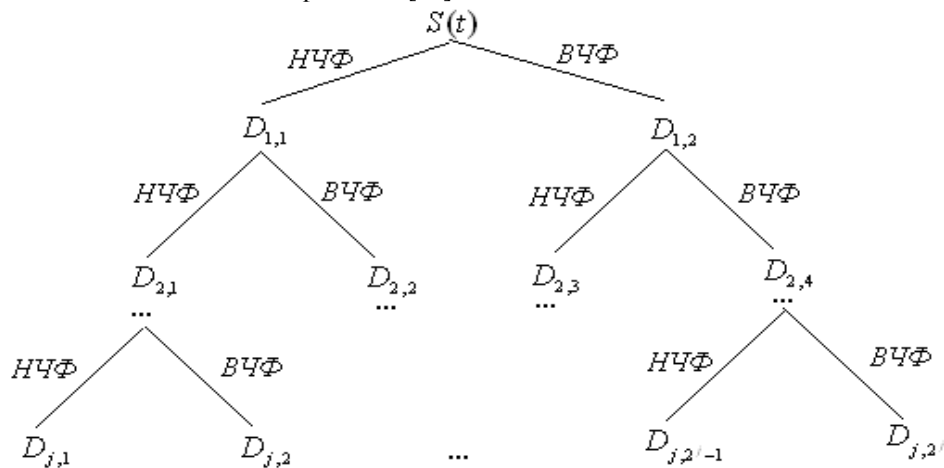
Рис.2 Дерево декомпозиції при пакетному вейвлет-перетворенні
