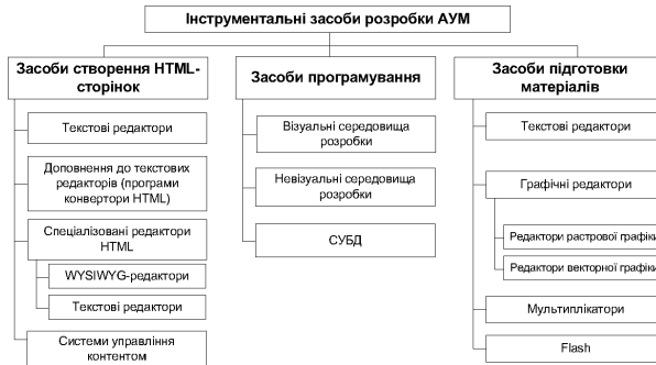
Рис. 2 – Класифікація інструментальних засобів розробки АУМ
