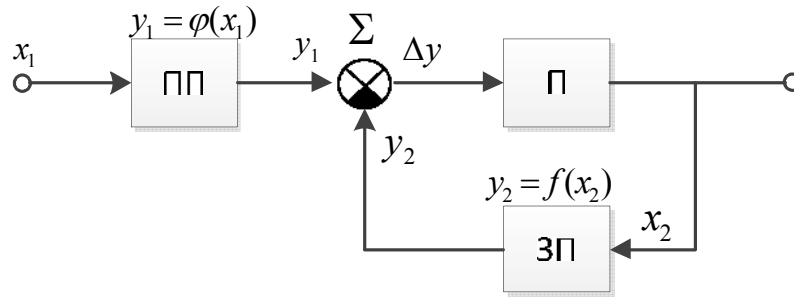
Рис. 1. Схема лінійного перетворювача зі зворотним зв'язком
