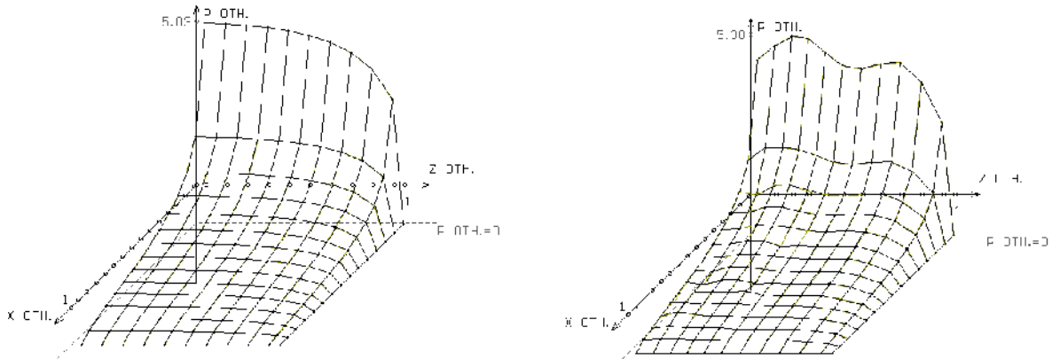
Рис. 8. Графік розподілу тиску по профілю прямого та хвилеподібного крил
