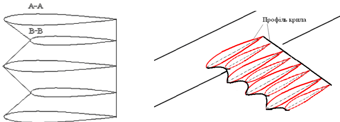
Рис. 1. Схематичне зображення моделі крила із хвилеподібною формою передньої кромки
