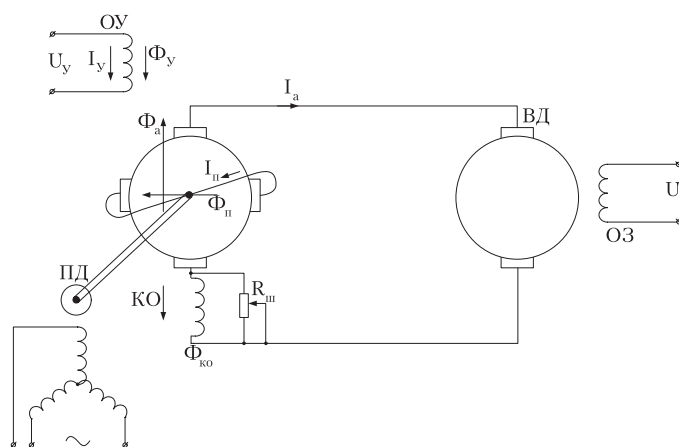
Рис. 1. Принципова схема включення ЕМП й двигуна постійного струму з незалежним збудженням
