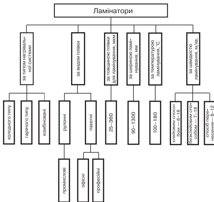
Рис. 2. Класифікація ламінаторів
