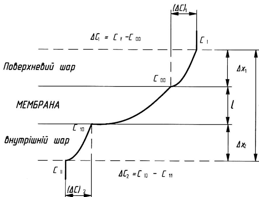
Рис. 2. Профіль концентрації рідини, що проникає через мембрану, в самій мембрані та в при мембранних прошарках: \Delta x_1 , \Delta x_2 - ефективна товщина при мембранних прошарків по обидві сторони мембрані, l - товщина мембрани; (\Delta c)_1 , (\Delta c)_2 - зміна концентрації в дифузійних шарах; c_1 , c_{11} - концентрація проникаючої через мембрану рідини в глибині розчинів, розділених мембраною. Пунктирна лінія – дійсний профіль зміни концентрації в при мембранних просторах
