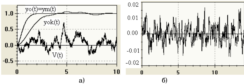
Рис. 7 – Результат дії випадкової завади
