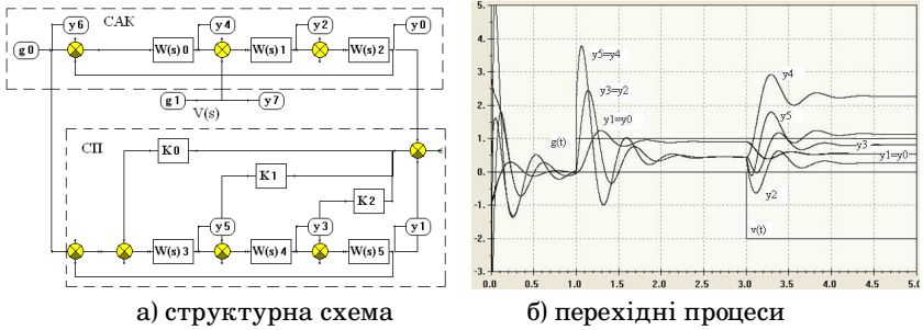
Рис. 1 – Спостерігач стану
