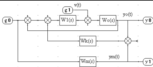
Рис. 3 – Одномірна система із еталоном-спостерігачем
