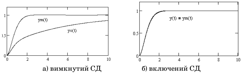
Рис. 4 – Перехідні процеси
