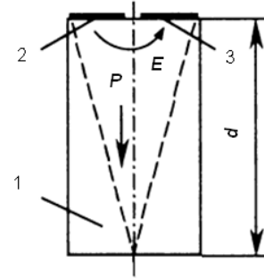
Рис. 4. Поверхнево збуджуваний товстий п'єзоперетворювач.
