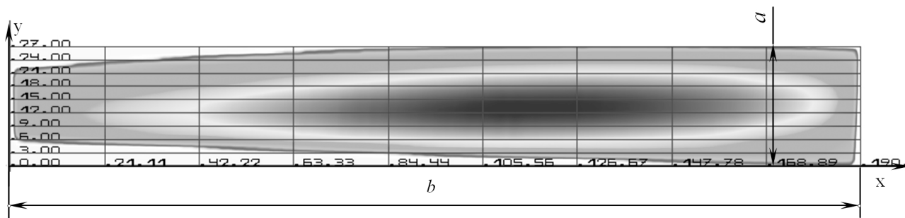
Рис. 3. Площадка контакта и распределения контактных давлений на входе в зацепление зубьев
