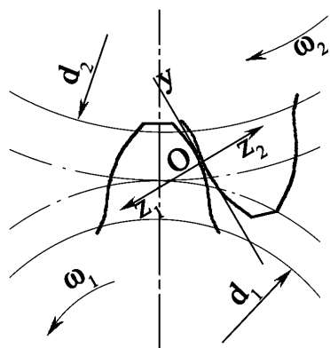
Рис. 1. Контакт двух зубьев зубчатых колес
