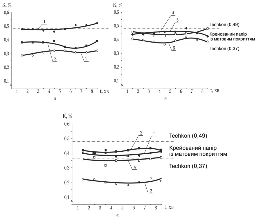
Рис. 3. Кінетика зміни загального контрасту зображення (закінчення) тиражного відбитка у межах процесу друкування для некрейдованого паперу масою 1 \text{ м}^2 120 \text{ г} (д, е) та для крейдованого хром-ерзацу масою 1 \text{ м}^2 280 \text{ г} (е). Режими кольороподілу: 1 — UCR; 2 — GCR None; 3 — GCR Maximum; 4 — GCR Light; 5 — GCR Medium; 6 — GCR Heavy
