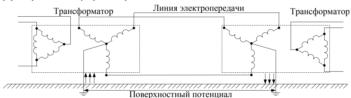
Рис.1. Воздействие поверхностного потенциала на электрическую сеть
