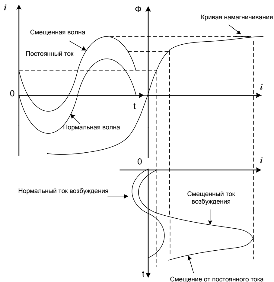
Рис.2. Смещение рабочей точки магнитной системы трансформатора
