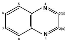
Fig. 1. Quinoxaline.
