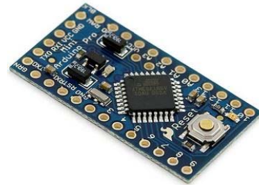
Figure 4 – Arduino Pro Mini micro-controller board.
