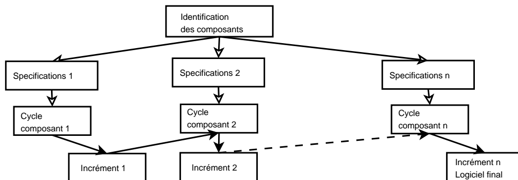
FIG. 3.3 – Cycle de vie Incrémental
