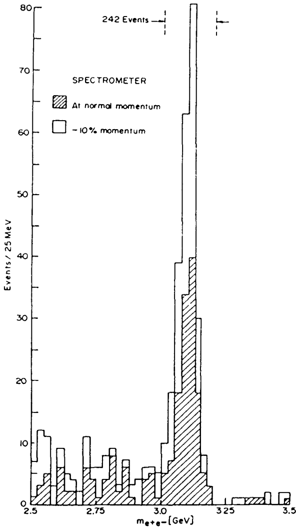
Fig. 1 Le J/\psi découvert comme pic dans la masse invariante de paires e^+e^- produites en collisions hadroniques.
