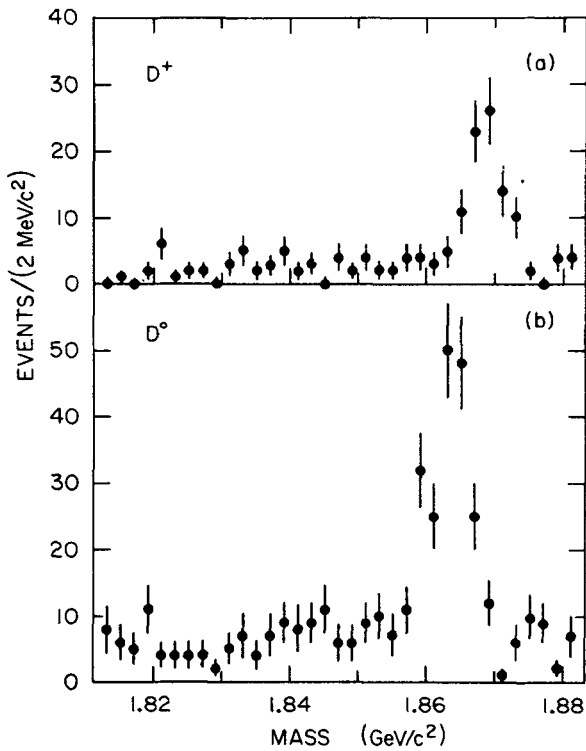
Fig. 7 Spectre de masses montrant les mesons D: D^+ dans la combinaison K^-\pi^+\pi^+ , D^0 dans la combinaison K^\pm\pi^\mp .
