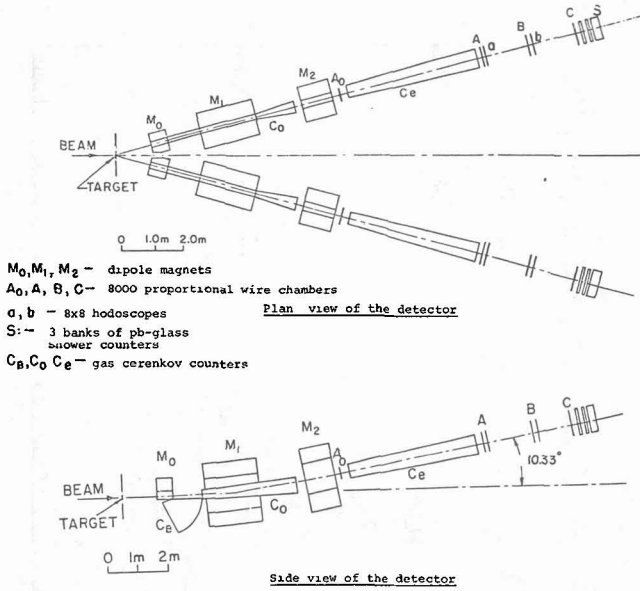
Fig. 3 Schéma du bispectromètre ayant mis en évidence le J/\psi à Brookhaven.
