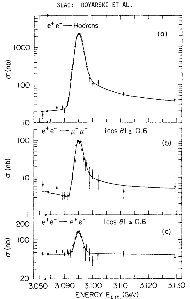
Fig. 2 Le J/\psi découvert comme pic dans la section efficace de la réaction e^+e^- \rightarrow \text{hadrons} .
