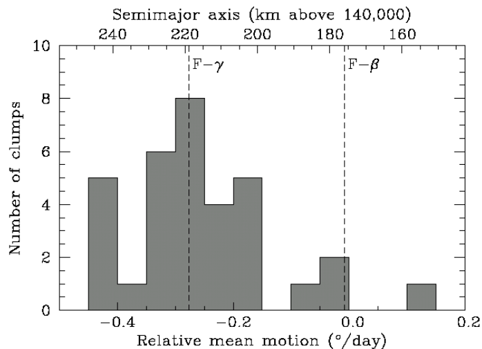
Figure 3.9 – Variation de la vitesse relative des clumps par rapport au mouvement moyen nominal de 582,27 \text{ }^\circ \cdot \text{jour}^{-1} . Une grande majorité des grumeaux ont un mouvement moyen comparable à celui de la strand \gamma ou cœur, tiré de (Showalter, 2004).
