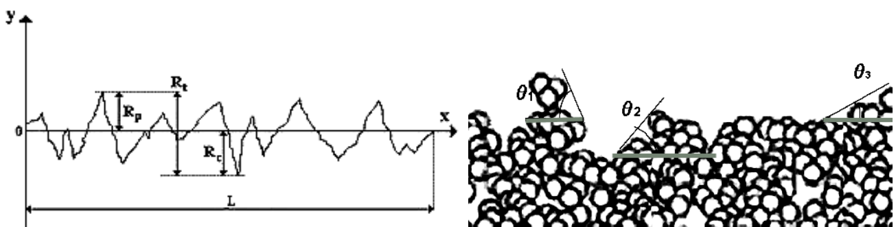
Figure 7.13 – Représentation schématique d'une rugosité définie par les longueurs et la rugosité de Hapke (1986) définie par des angles. R_c , R_p et R_t = |R_p + R_c| ainsi que \theta sont définis dans le texte.
