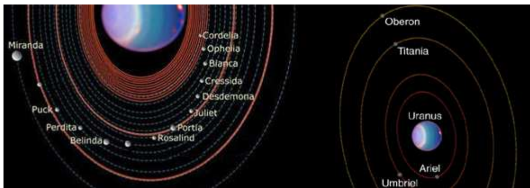
Figure F.10 – L'écosystème d'Uranus (♅)
