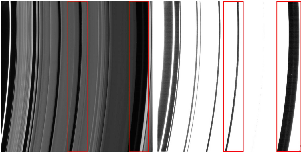
Figure D.11 – Images N1536485050 et N1504 faisant apparaître les annelets 1,971 R_5 et 1,988 R_5 dans la Division de Cassini
