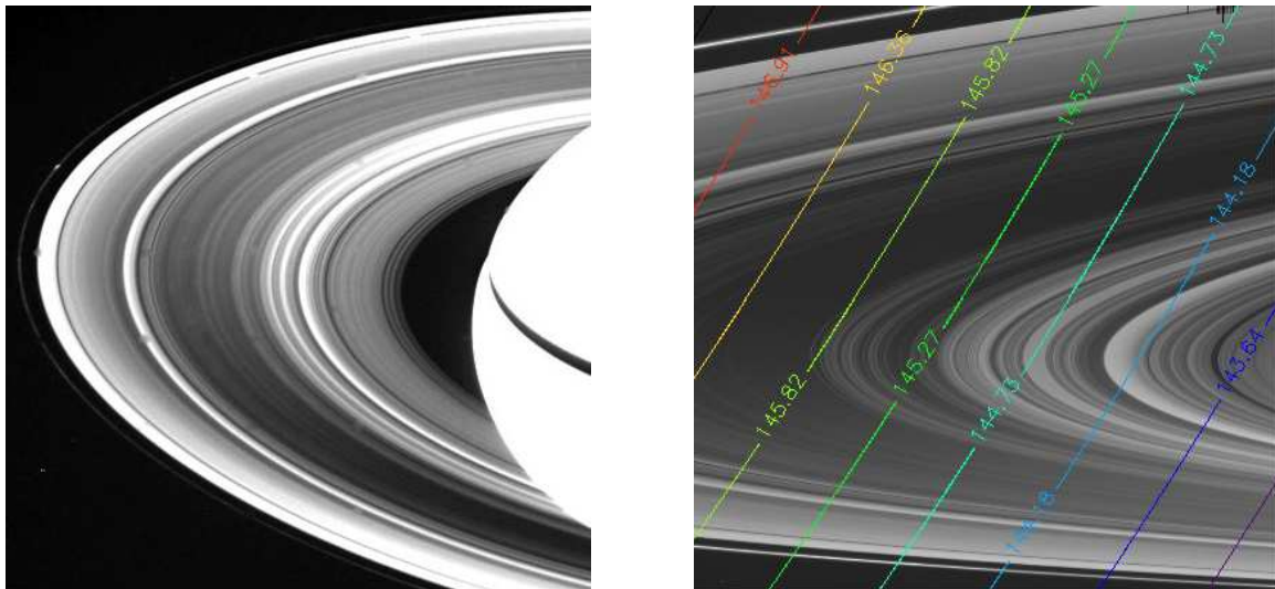
Figure C.4 – A gauche – Image VOYAGER faisant clairement apparaître la lumière diffusée de Saturne par les anneaux (PIA01955). Il suffit de regarder par exemple l'anneau B en haut de l'image : il est beaucoup plus brillant qu'en bas à droite où la diffusion de la lumière de Saturne par les anneaux est moins importante. A droite – Image CASSINI faisant apparaître le même phénomène (W1477669029). Les isocontours d'angles de phase sont indiqués et montrent bien qu'il ne s'agit pas d'un simple effet de phase.
