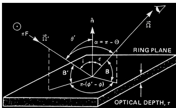
Figure E.2 – Paramètres géométriques : \pi F est le flux solaire incident en \text{W.m}^{-2} , i=\theta' est l'angle d'incidence, \epsilon=\theta est l'angle d'émission, \alpha \neq i+\epsilon est l'angle de phase et \Theta=\pi-\alpha l'angle de diffusion. B et B' sont les angles d'élévation de l'observateur et du Soleil. \phi est l'angle d'azimut. La normale à la surface est \hat{n} . Tiré de [Cuzzi et al. , 1984].
