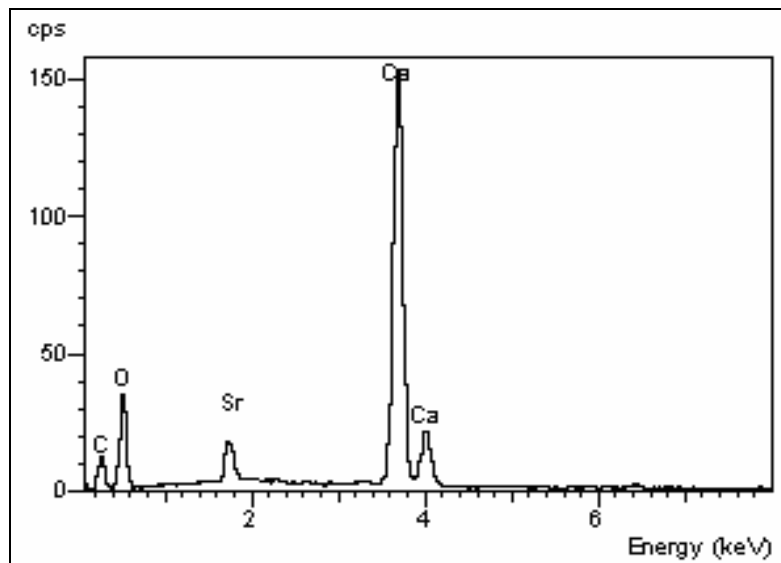
Figure 32 : Spectre d'émission d'énergie de l'échantillon A12. Quatre éléments chimiques apparaissent : le carbone, l'oxygène, le calcium et le strontium. Ce dernier substitue une partie des atomes de calcium dans le réseau cristallin de l'aragonite
