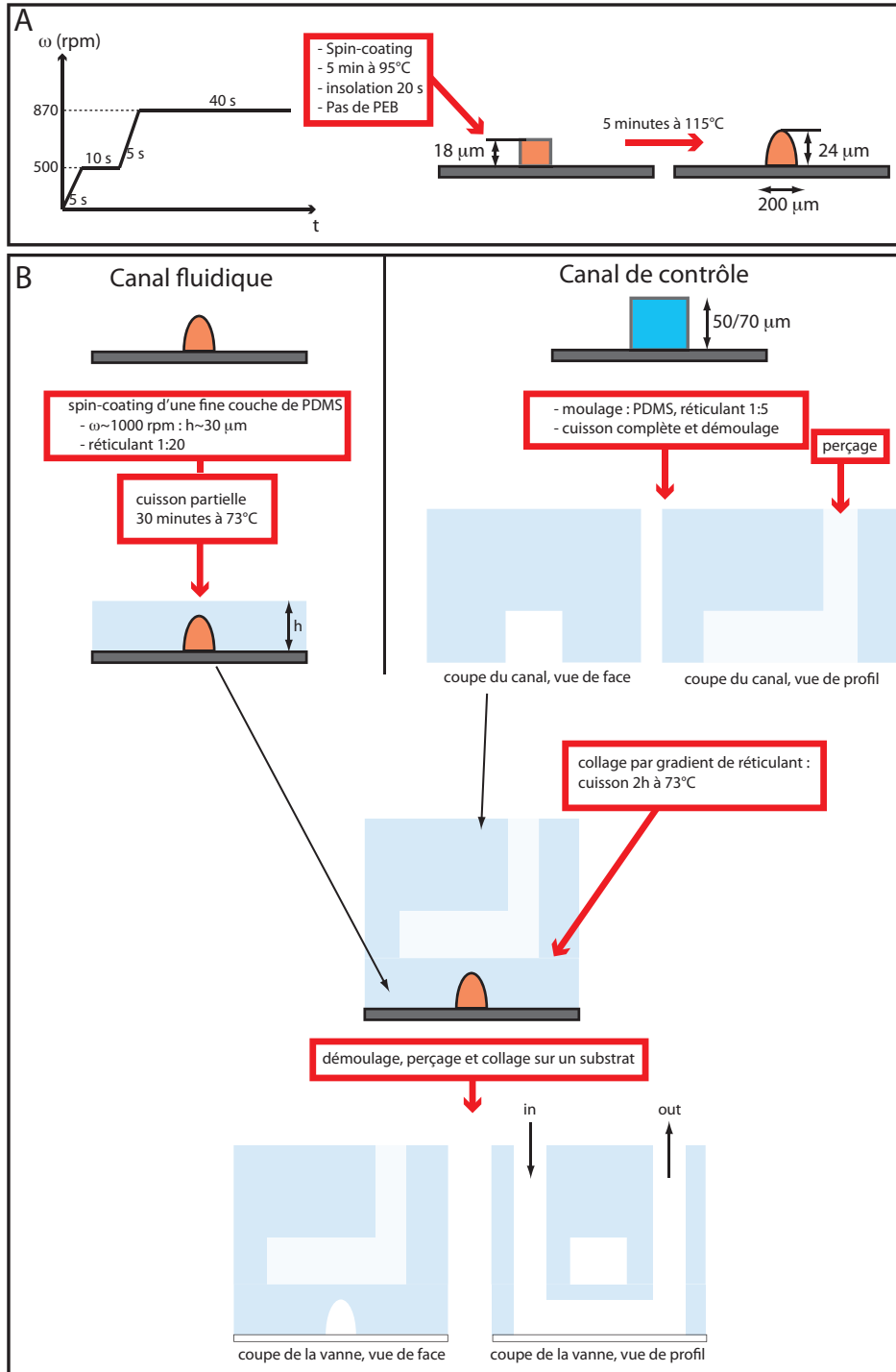
Fig. B.1: Fabrication des vannes. Les schémas ne sont pas à l'échelle. A : Protocole de lithographie pour la résine positive. Une dernière étape de cuisson modifie la forme des canaux. B : Lithographie multicouche, avec collage par gradient de réticulation. L'entrée du canal fluide (in) est ensuite connectée au réservoir de fluide, et la sortie (out) au canal d'étude.
