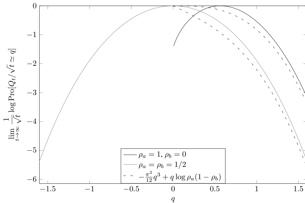
FIGURE 5.2 – Fonction de grande déviation rescalée G(q) du courant Q_t pour un processus d'exclusion symétrique sur la ligne infinie, pour \rho_a = 1 , \rho_b = 0 et pour \rho_a = \rho_b = 1/2 . La fonction G(q) , qui peut être obtenue numériquement par transformée de Legendre à partir de la fonction génératrice \log \langle e^{\lambda Q_t} \rangle_{\rho_a, \rho_b} (4), se rapproche rapidement de son expression asymptotique pour q \gg 1 (5.17).
