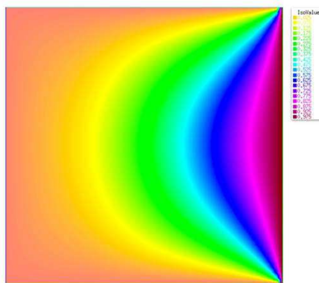
FIGURE 4.6: Dérivée par rapport à a de la solution du problème de Poisson 4.30 avec bord variable.
