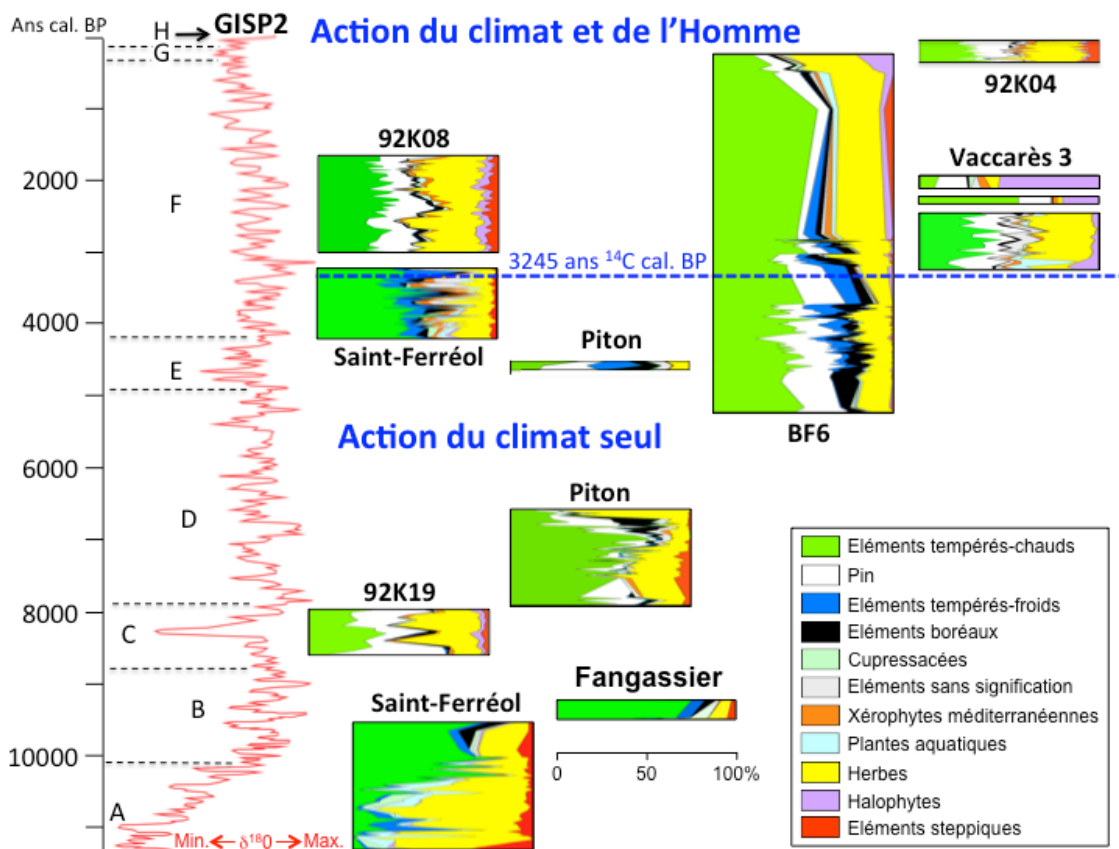
Fig. 7. Diagrammes polliniques 52 synthétiques des carottes réécemment étudiées 53 , corrélées avec la courbe isotopique de l'oxygène GISP2 de Grootes et Stuiver 54 , calibrée en années cal. BP, sur laquelle les grandes phases climatiques (A à H) ont été situées. La localisation des carottages se trouve sur la fig. 6A.
