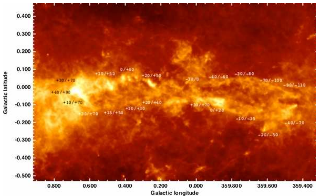
FIGURE 9.5 – Cartes en densité de colonne de la Zone Moléculaire Centrale pour l \in [-0.75^\circ, +0.87^\circ] et b \in [-0.5^\circ, +0.5^\circ] issue de l'observation à 250 \mu\text{m} par le télescope SPIRE de l'observatoire Herschel.
