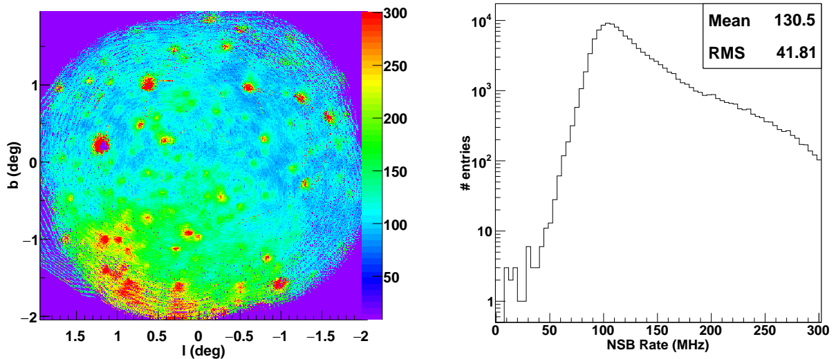
FIGURE 10.7 – Taux de bruit de fond du ciel issu de l'analyse des distributions de piédestaux de la chaîne de haut gain pour les pixels de la caméra de CT5. A gauche, distribution du taux de NSB sur le champ de vue (en coordonnée galactique). A droite, projection de cette distribution.
