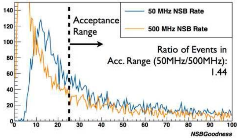
FIGURE 8.12 – Distribution de NSB Goodness en intensité pour des photons simulés avec un taux de NSB de 50 MHz (en bleu) et de 500 MHz (en jaune). Figure produite par M. Holler.
