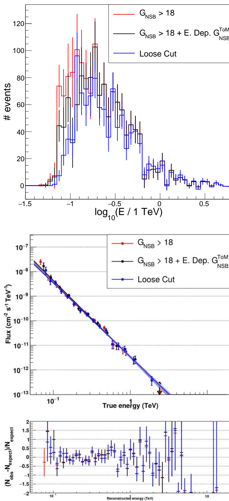
FIGURE 8.20 – Distributions de l'énergie reconstruite et spectres ajustés par une loi de puissance issus des analyses monoscopiques de PKS 2155-304. En bleu, coupure Loose . En rouge, coupure G_{\text{NSB}} > 18 . En noir, coupure G_{\text{NSB}} > 18 + \text{E. Dep. } G_{\text{NSB}}^{\text{ToM}} .
