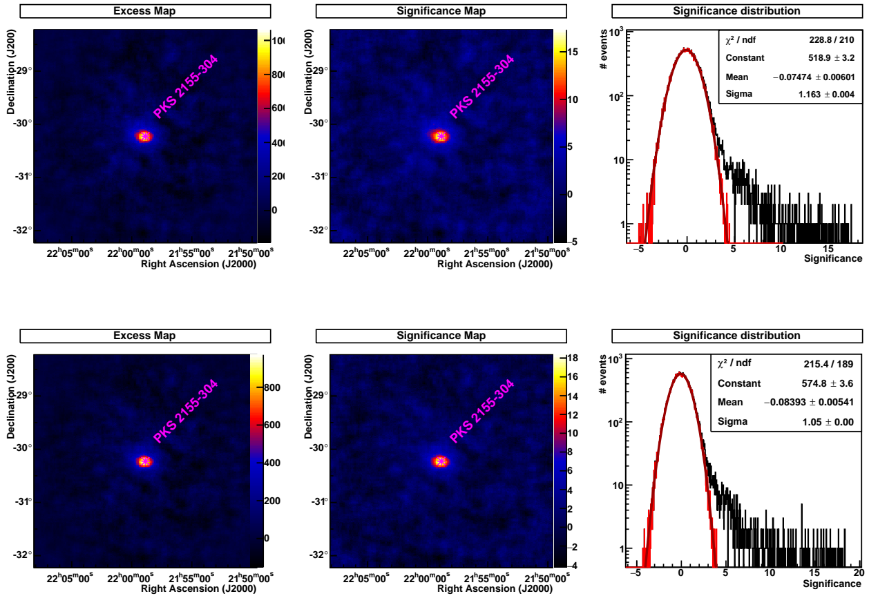
FIGURE 8.18 – Cartes en excès d'événements (à gauche) et en significativité (au centre) issues de l'analyse monoscopique de la région de PKS 2155-304. A droite, distribution de la significativité de la source en noir ( 0.4^\circ autour du centre de l'image) et du fond en rouge sur laquelle est ajustée une fonction gaussienne (en rouge foncé).
