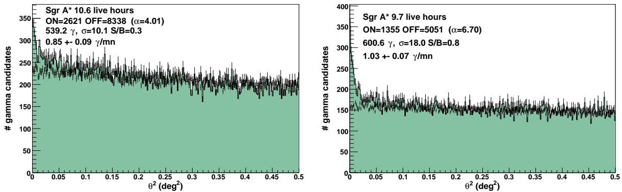
(b) Analyses monoscopique (à gauche) et stéréoscopique (à droite) avec les coupures Loose .
