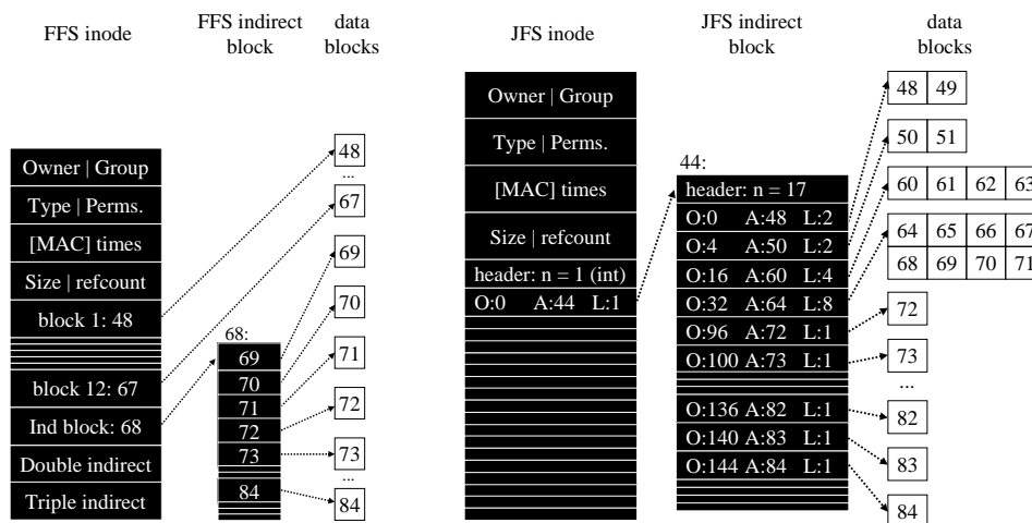
Abbildung 1: Vergleich der zur Dateiallokierung eingesetzten Datenstrukturen
