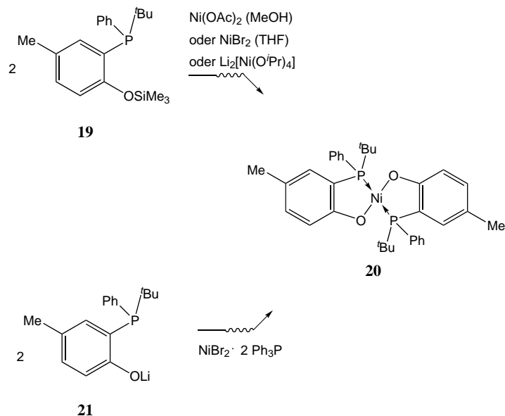
Schema 3.4: Synthesewege des trans-konfigurierten Nickel-Chelat-Komplexes 20 .
