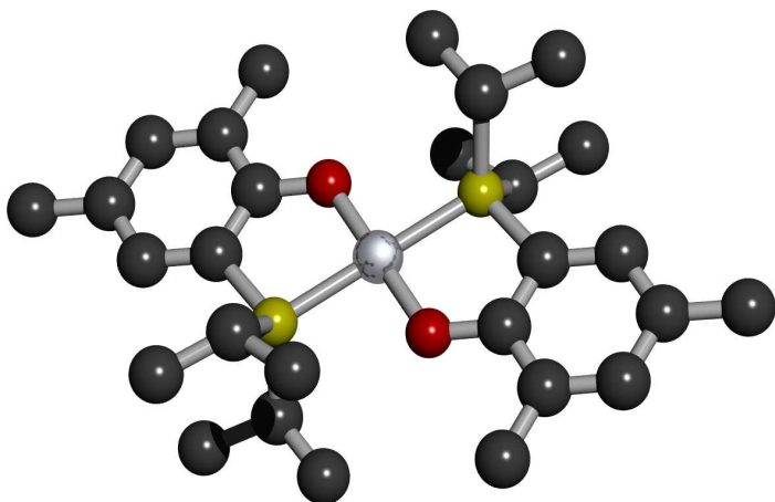
Abbildung 3.6: Röntgenstruktur des trans-konfigurierten i Pr/ i Pr-Komplexes 24 [9].
