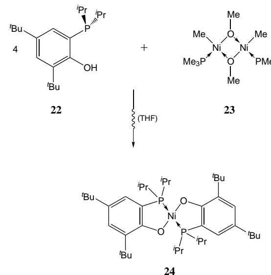
Schema 3.5: Synthesewege des trans-konfigurierten Nickel-Chelat-Komplexes 24.
