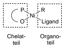
Abbildung 3.1: Allgemeine Form der Katalysator-Vorstufe beim SHOP.
