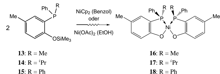
Schema 3.3: Darstellung von cis-konfigurierten Nickel-Chelat-Komplexen.
