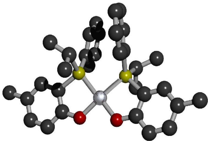
Abbildung 3.5: Röntgenstruktur des cis-konfigurierten i Pr/Ph-Komplexes 17 [8].
