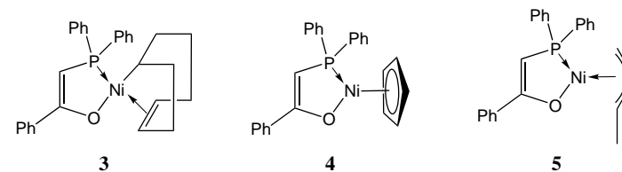
Abbildung 3.2: Beispielverbindungen für Katalysator-Vorstufen für den SHOP [3].
