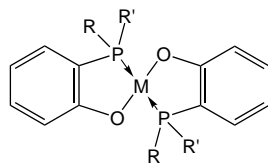
Abbildung 3.3: Allgemeine Struktur der trans-konfigurierten Bis(2-phosphanylphenolato)-Chelatkomplexe
