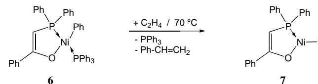
Schema 3.2: Bildung eines SHOP-Katalysators [3]
