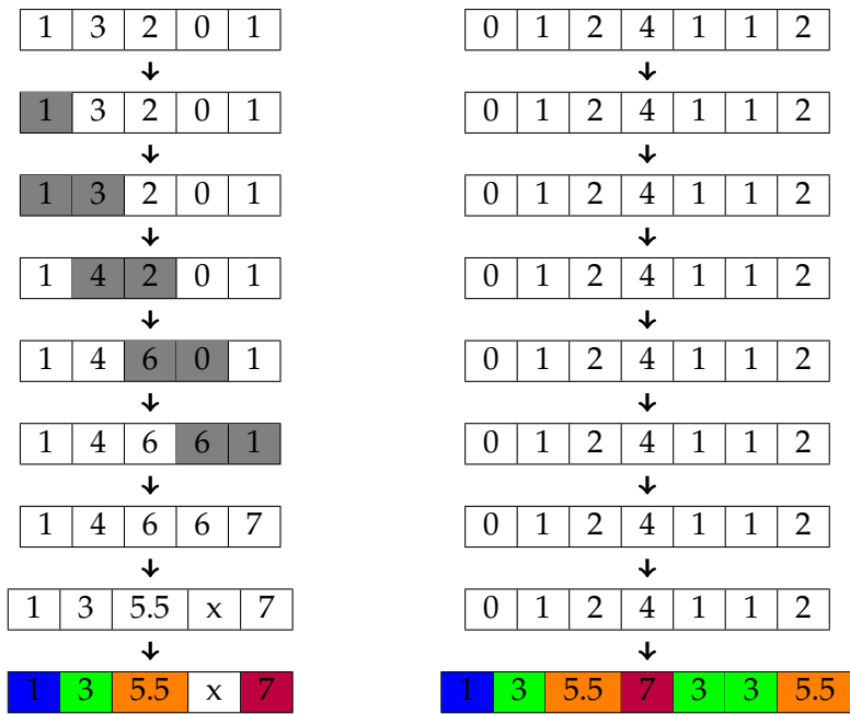
FIGURE 3.6 – Calcul des rangs pour l’ensemble \{0, 1, 2, 4, 1, 1, 2\} pas à pas.
