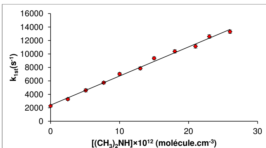
Graphique du second ordre pour la réaction CN + (CH_3)_2NH à 36.1 K dans Hélicum [He]= 5.28 \times 10^{16} \text{ cm}^{-3}
