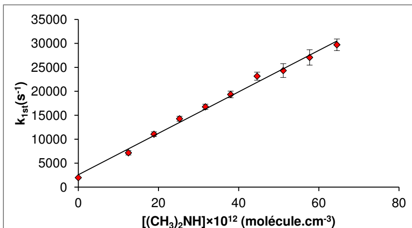
Graphique du second ordre pour la réaction \text{CN} + (\text{CH}_3)_2\text{NH} à 49.1 K dans Hélium [\text{He}] = 10.4 \times 10^{16} \text{ cm}^{-3}
