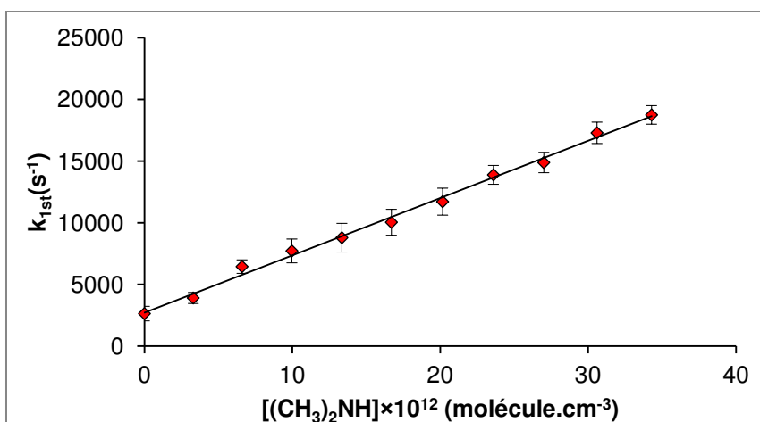
Graphique du second ordre pour la réaction CN + (CH_3)_2NH à 22.9 K dans Hélicum [He]= 4.73 \times 10^{16} \text{ cm}^{-3}
