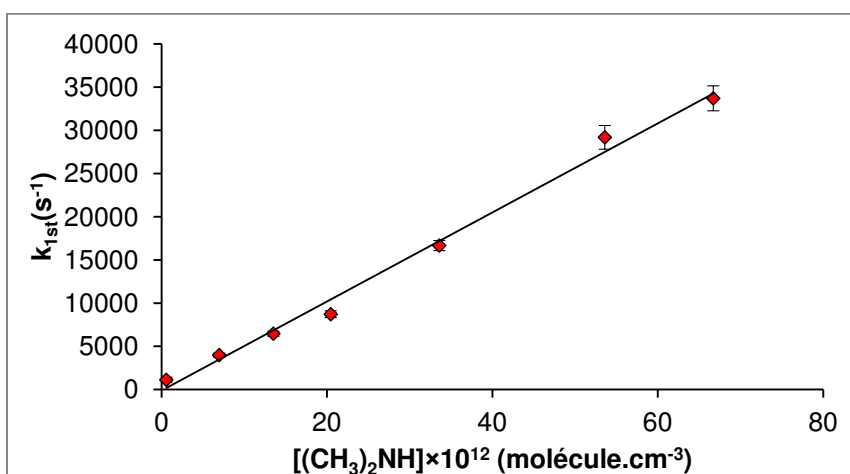
Graphique du second ordre pour la réaction \text{CN} + (\text{CH}_3)_2\text{NH} à 71.6 K dans Hélium [\text{He}] = 6.01 \times 10^{16} \text{ cm}^{-3}
