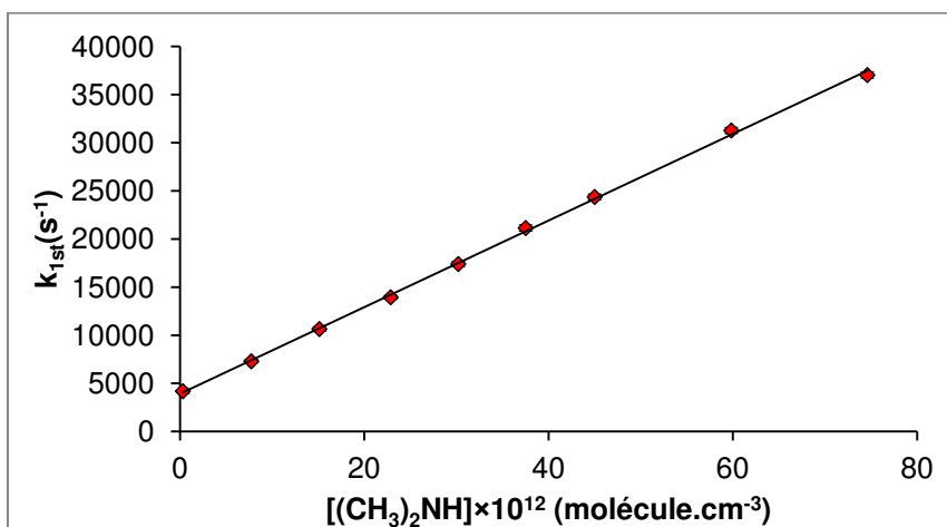
Graphique du second ordre pour la réaction \text{CN} + (\text{CH}_3)_2\text{NH} à 123 K dans Hélium [\text{He}] = 12.7 \times 10^{16} \text{ cm}^{-3}
