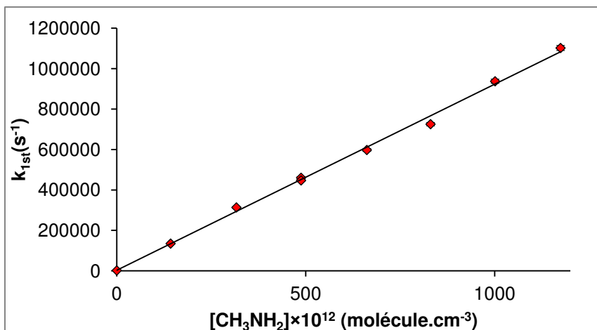
Graphique du second ordre pour la réaction CN + CH_3NH_2 à 297 K dans Hélicum [He]= 13.55 \times 10^{16} \text{ cm}^{-3}
