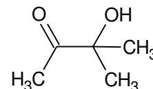
3-hydroxy-3-méthyl-2-butanone
