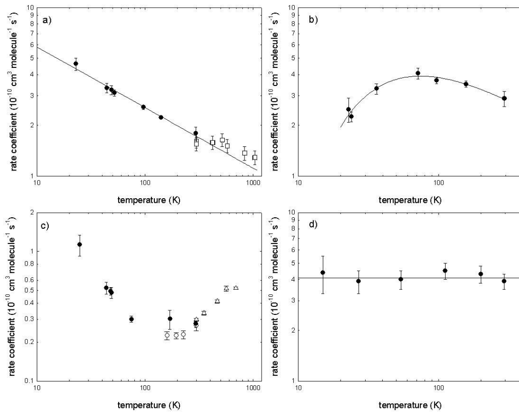
Figure 1.4 : Constantes de vitesse des r actions a) Al + O 2 , b) B + Ac tyl ene, c) CN+ C 2 H 6 d) CN + Propadi ene en fonction de la temp erature. Les cercles noirs repr esentent les valeurs mesur es   l'aide de la technique CRESU et les autres symboles dans a) et c) repr esentent des valeurs obtenues dans la litt erature par Garland et al. 54 , Hebert et al. 55 et Sims et al. 56 .
