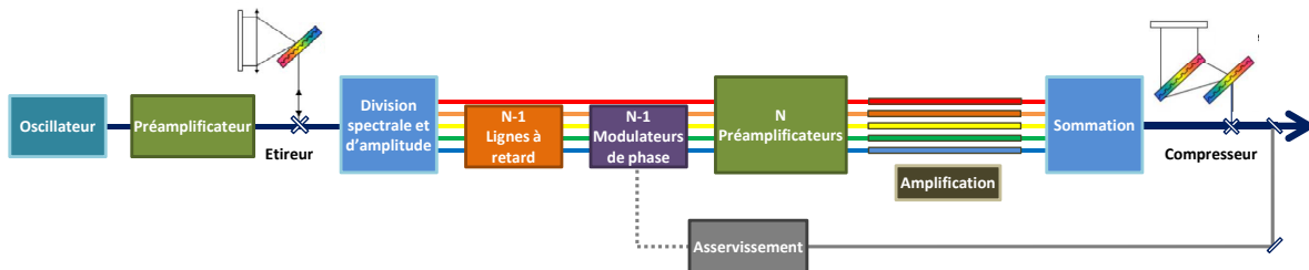
FIGURE III-28 : Proposition de schéma de combinaison cohérente spectrale stabilisée par voie active à N voies.
