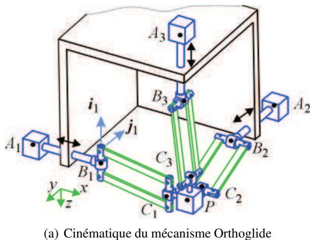
FIGURE 1.9 – Mécanisme isotrope à trois degrés de liberté Orthoglide
