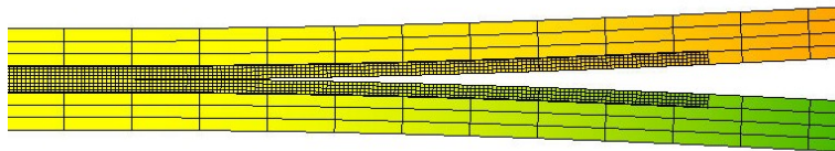
Figure 4.28 — Maillages des deux modèles pour l'essai DCB en 2D.
