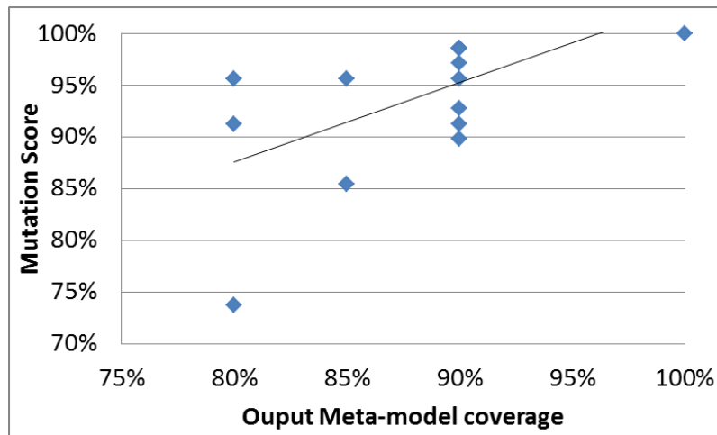
(a) Oracles utilisant des modèles attendus
