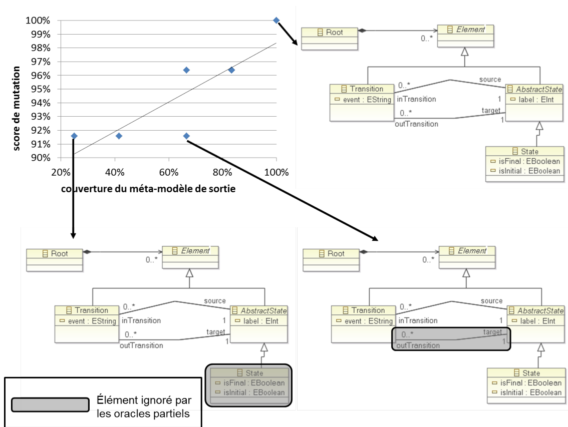
Figure 4.11 – Taux de couverture et score de mutation pour la transformation f_{sm2ffsm} (modèles attendus)
