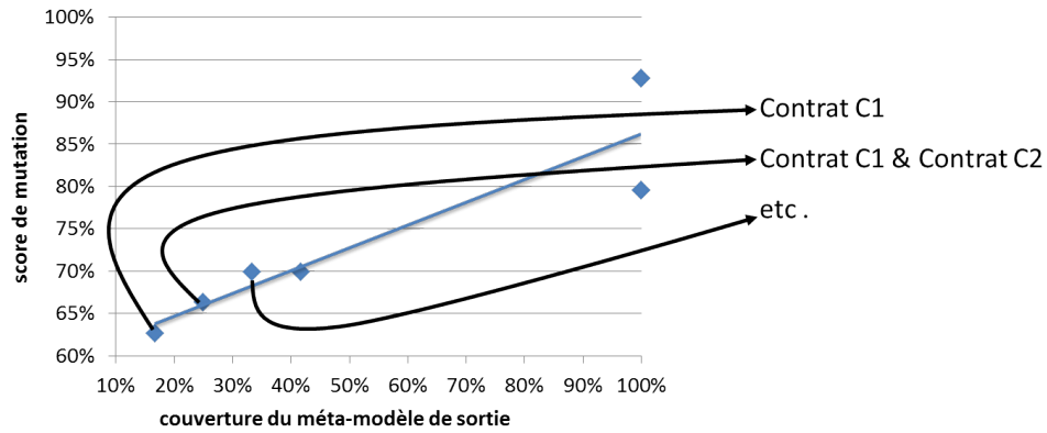
Figure 4.13 – Taux de couverture et score de mutation pour la transformation f_{sm2ffsm} (contrats incrémentaux)
