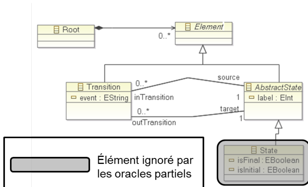
Figure 4.9 – Éléments couverts par l'ensemble d'oracles P1
