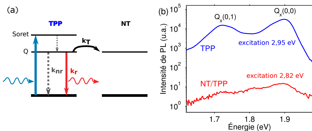
FIGURE 5.9 – (a) Schéma de relaxation de la TPP après excitation de la bande de Soret. Les mécanisme envisagés sont un transfert vers les nanotubes ( k_T ), une recombinaison radiative ( k_r ) ou non radiative ( k_{nr} ). (b) Spectre de photoluminescence des solutions de TPP libres (bleu) et NT/TPP (rouge), sous excitation avec leur bande de Soret respective à 2,95 eV et 2,82 eV.
