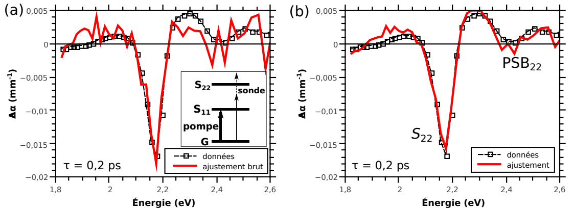
FIGURE 3.24 – Spectre d’absorption transitoire (carrés noirs) ajusté par déformation du spectre complet (ligne rouge) pour une pompe résonante avec S_{11} de flux 3,2 \cdot 10^{14} photons. \text{cm}^{-2} photons pour un retards de 0,2 ps. L’ajustement est effectué directement (a) ou en effectuant la procédure décrite dans le texte pour N = 4 (b).
