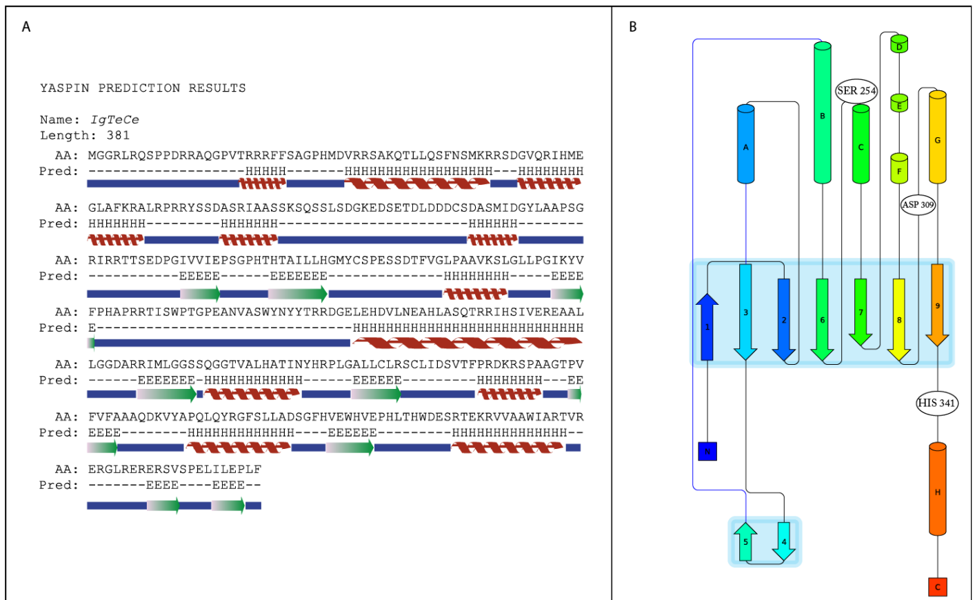
Figure 34: Prédications de la structure secondaire d' IgTeCe
