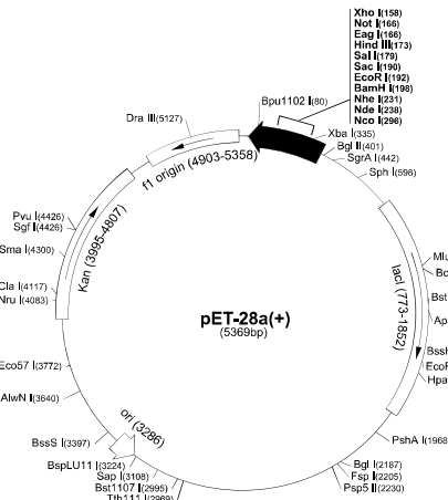
Figure 23: Le vecteur d'expression pET28a+
