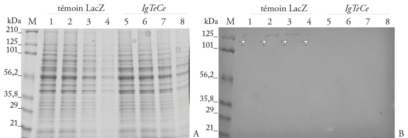
Figure 44: A) Electrophorèse sur SDS-PAGE 12 % des extraits protéiques déposés pour le Western blot. B) Western blot des extraits protéiques.
