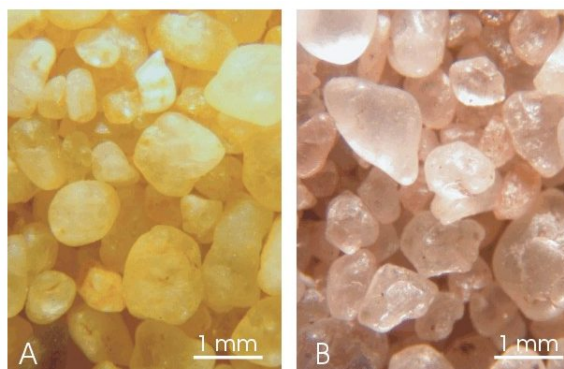
FIGURE 1.29 – Propriétés physiques des grains indiquant des agents de transport différents. A. Sable quartzueux éolien dont les grains ont un aspect “ rond-mat ” indiquant une érosion par le vent, B. sable quartzueux dont les grains ont un aspect “ émoussé-luisant ” indiquant une érosion par l’eau. (Credit : http://www2.ulg.ac.be/ )
