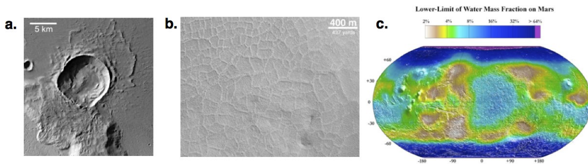
FIGURE 1.6 – Témoins d’un pergélisol dans le sous-sol martien. (a) Cratères à éjecta lobé (credit : ESA/DLR/FU Berlin), (b) polygones de contraction thermique (image MOC/MGS) (credit : NASA/JPL/MSSS/ASU), (c) carte de la teneur en eau équivalent obtenue à partir des données GRS/Mars Odyssey ( Feldman et al. , 2004) (credit : NASA/JPL/Los Alamos National Laboratory).
