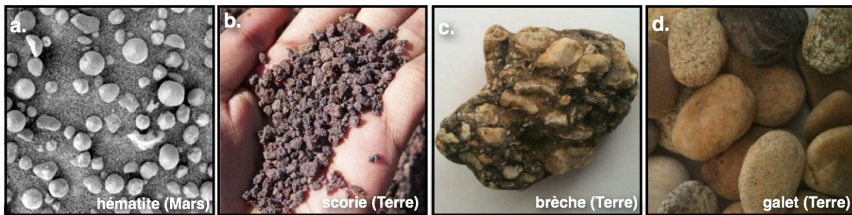
FIGURE 1.22 – Exemples d’échantillons avec des formes et rugosités variées. a. sphérules d’hématites sur Mars (1 mm de diamètre), b. scories d’Auvergne avec une rugosité vacuolaire (5 mm de diamètre), c. brèche (environ 10 cm) avec des éléments angulaires et d. galets de forme arrondie et plate (5 cm de diamètre).
