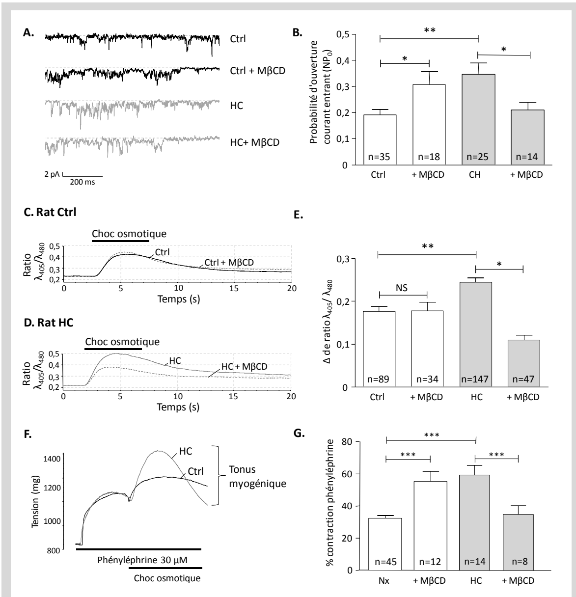
Figure 59 : A. Exemples de courants entrant par les SAC, en configuration cellule attachée, suite à un étirement de -40 mmHg, chez des rats Ctrl et HC, en présence ou en absence de M \beta CD (5 mM). B. Probabilité d'ouverture du courant unitaire entrant après un étirement. C et D. Exemple de traces calciques en indo-1 après un choc osmotique chez un rat Ctrl ( C ) et HC ( D ) en présence ou en absence de M \beta CD (5 mM). E. Amplitude du pic calcique après un choc osmotique. F. Exemple de trace de contraction mesurée dans des cuves à organe isolé après un choc osmotique chez un rat Ctrl et HC en présence de 2 mM de Ca 2+ extracellulaire. G. Pourcentage de la contraction au choc osmotique sur la précontraction à la phényléphrine (30 \mu M), en absence ou en présence de M \beta CD (5 mM).
