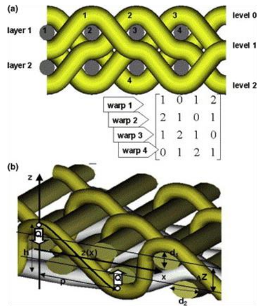
Figure 4-2. Exemple de structure tissée intégrée dans WiseTex : (a) Codage de l'armure tissée ; (b) description des trajectoires des fils [7].
