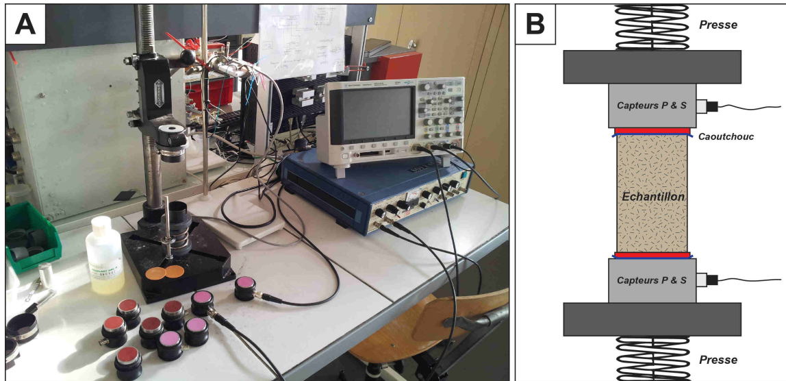
FIGURE 39 – A - Appareillage de mesure des vitesses de propagation d’ondes P & S. B - Détail du dispositif capteur-échantillon.
