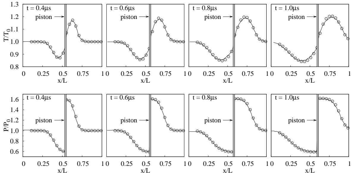
FIGURE 3.18 – Comparaison entre DSMC (—) et modèle BGK avec une approche maille coupée (⊙). Les profils de température (en haut) et de pression (en bas) sont tracés à quatre instants différents, et les conditions aux limites sont diffuses.
