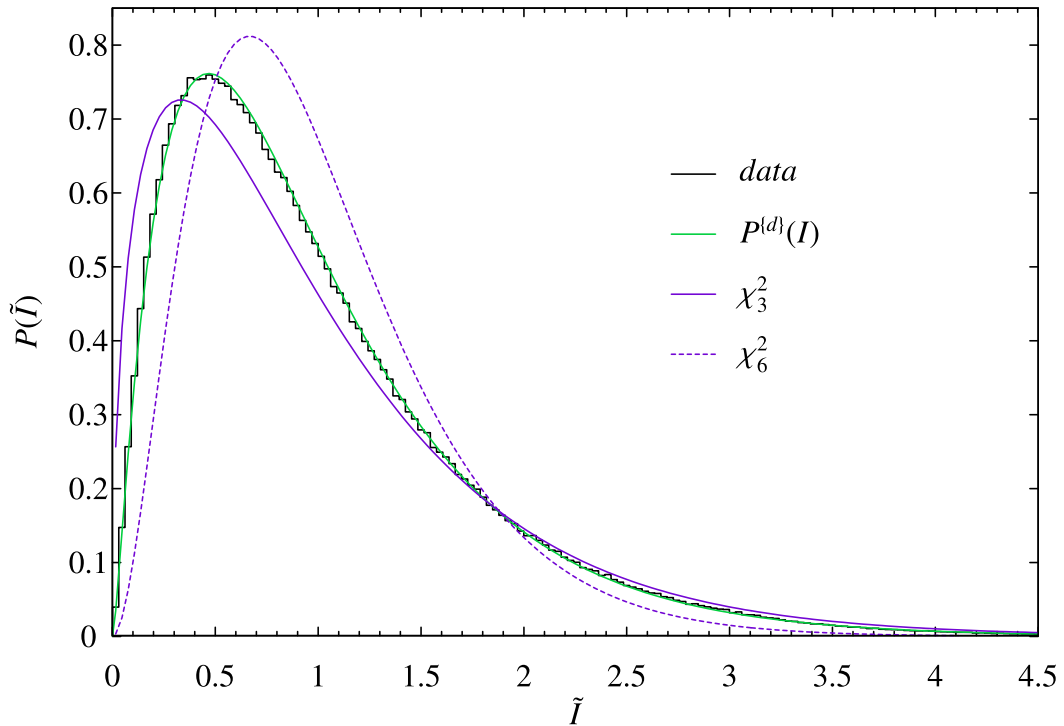
FIGURE 4.16 – Comparaison de la distribution d'intensité des réponses de la CR chaotique (Figure 4.3) avec la prédiction TMA P^{\{d\}} et les distributions attendues dans un système complètement fermé ( \chi_3^2 ), et dans un système complètement ouvert ( \chi_6^2 )
