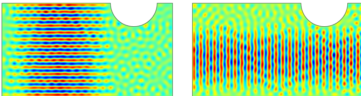
FIGURE 1.10 – Exemple de modes non-génériques de type bouncing ball dans un billard de Sinai 2D
