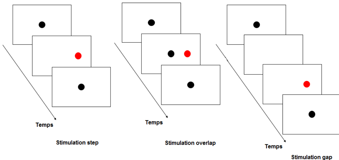
Figure 35: Paradigmes expérimentaux
