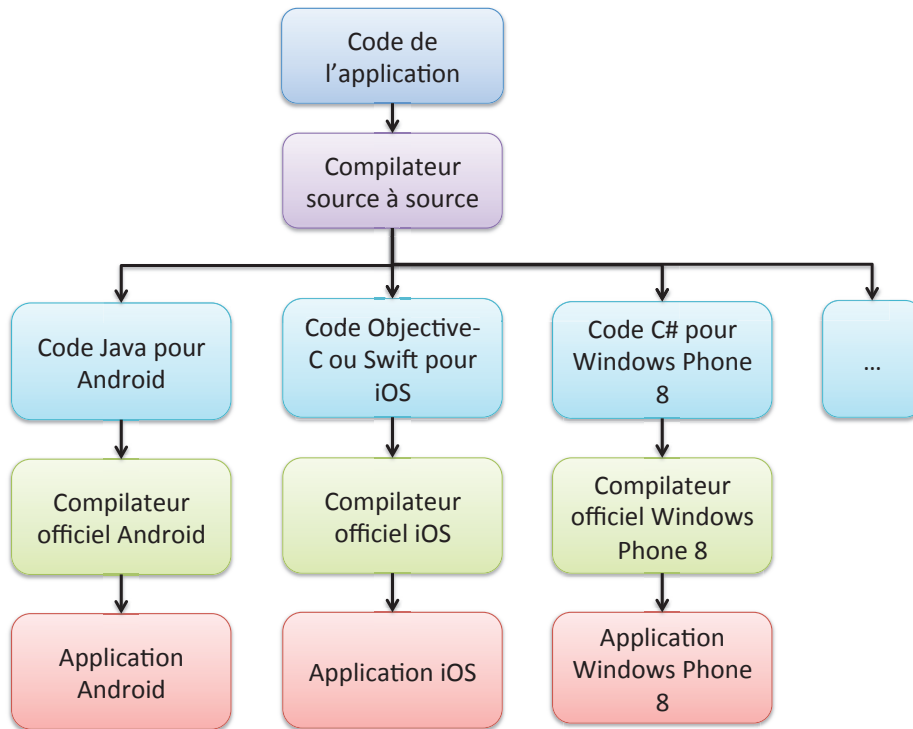
FIGURE 3.4 – Principe de la compilation source à source application au développement mobile multiplateforme
