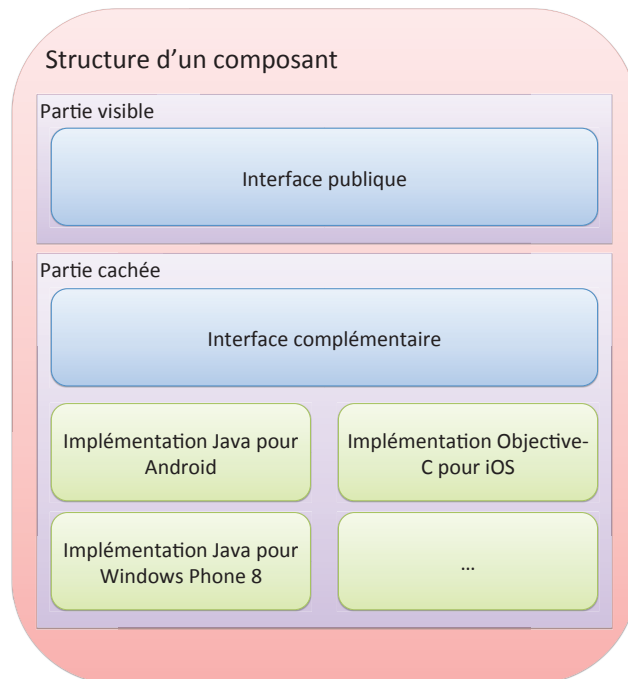
FIGURE 6.7 – Structure d'un composant multiplateforme dans notre solution
