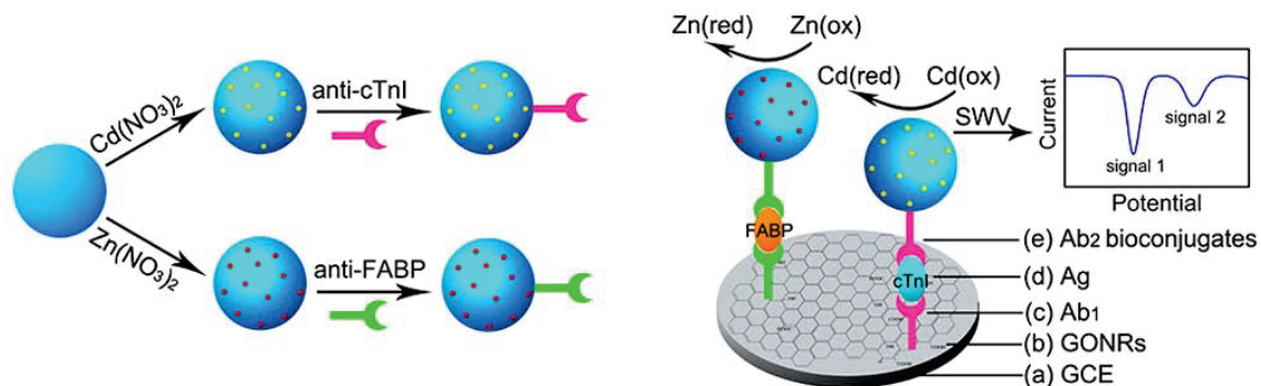
Figure 1-22. Stratégie de marquage par des nanoparticules métalliques pour la détection électrochimique d'interactions antigène/anticorps
