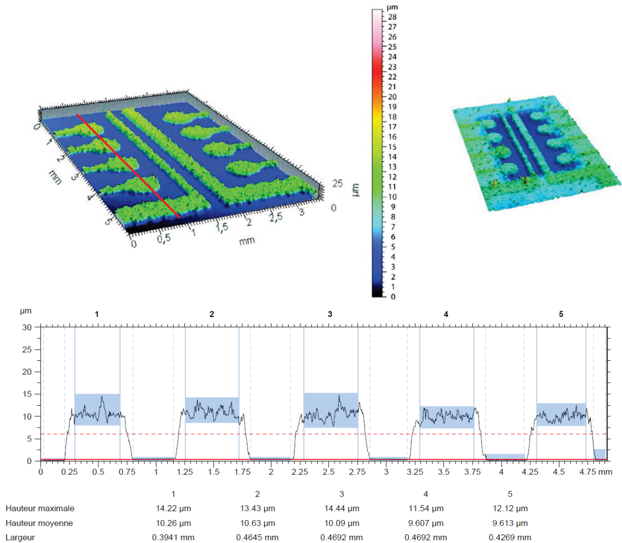
Figure 6-2. Image de profilométrie et profil du réseau d'électrodes
