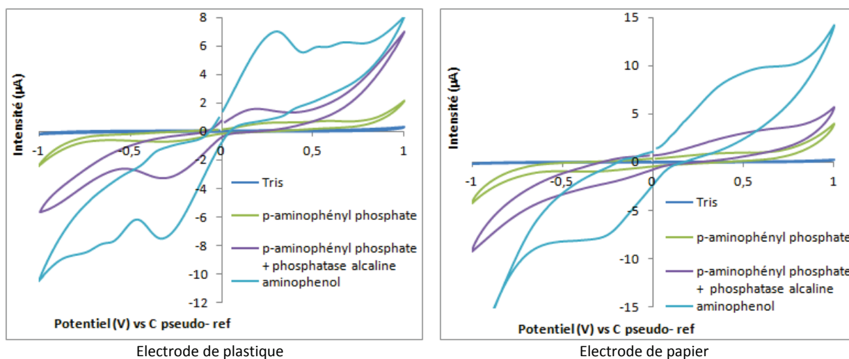
Figure 6-7. Courbes de voltammétrie cyclique en présence du substrat ou produit de la phosphatase alcaline
