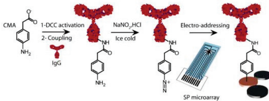
Figure 1-8. Electroaddressage d'anticorps modifiés sur la surface d'une électrode sérigraphiée (Extrait de Corgier et al. 2005) CMA : 4-carboxyméthylaniline ; DCC : N,N'-dicyclohexylcarbodiimide
